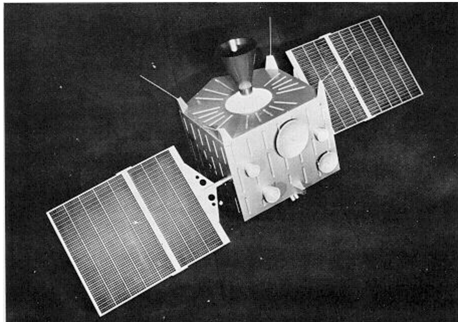
Fig. 13 — Maquette du satellite de télécommunications (version C) proposé à la CETS
